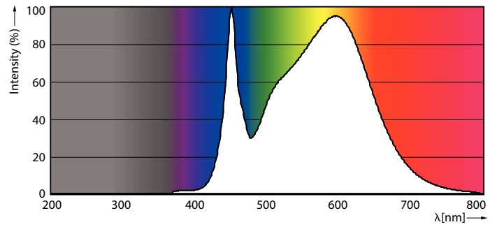
LEDtube 24W G13 3700lm 840
